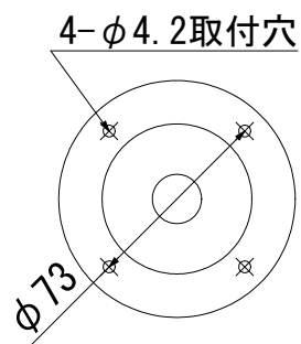
＜＜取付面 寸法図＞＞
