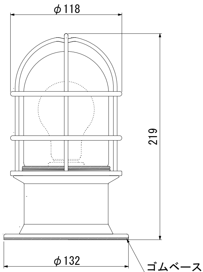
<<取付面 寸法図>>
