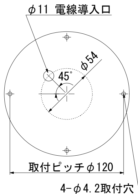
<<取付面 寸法図>>
