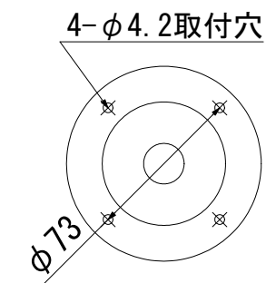
＜＜取付面 寸法図＞＞
